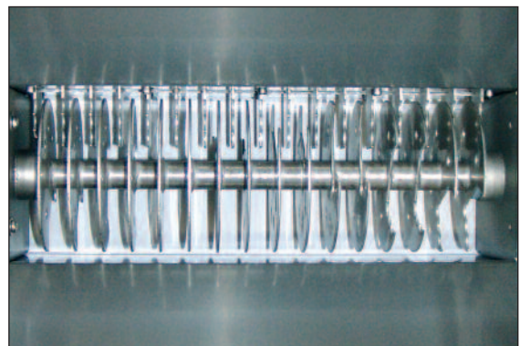
Mahlwerk des Crushermoduls aus solidem Edelstahl.
