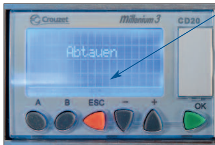
Die aktuellen Betriebszustände werden dem Anwender über das digitale Display in der Frontblende angezeigt
