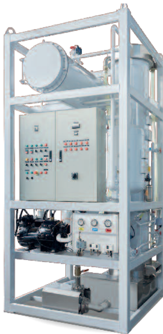
PATKOL-WESSAMAT-Eisbereitungsanlage Modell PK 10 AU
