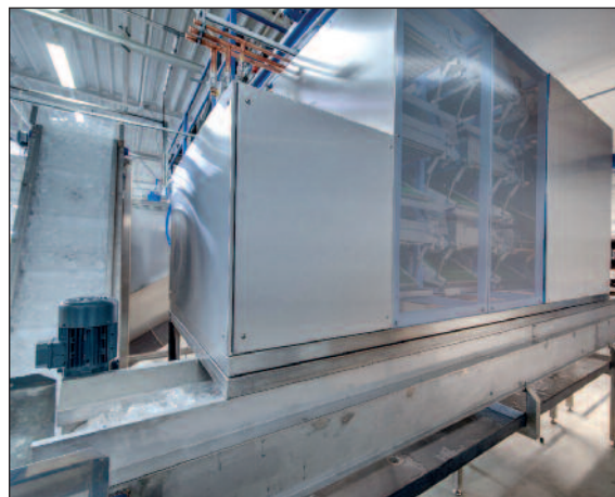
Eisbereitungsanlage IC 1500 auf Eistransportband zur Herstellung von quadratischen Volleiswürfeln
