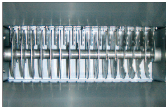
Mahlwerk des Crushermoduls aus solidem Edelstahl.
